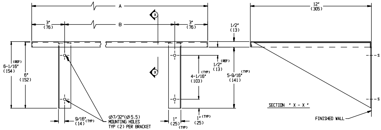
ELEVATION
