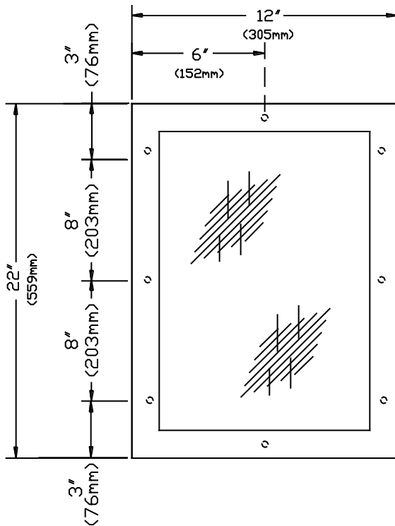
ELEVATION
